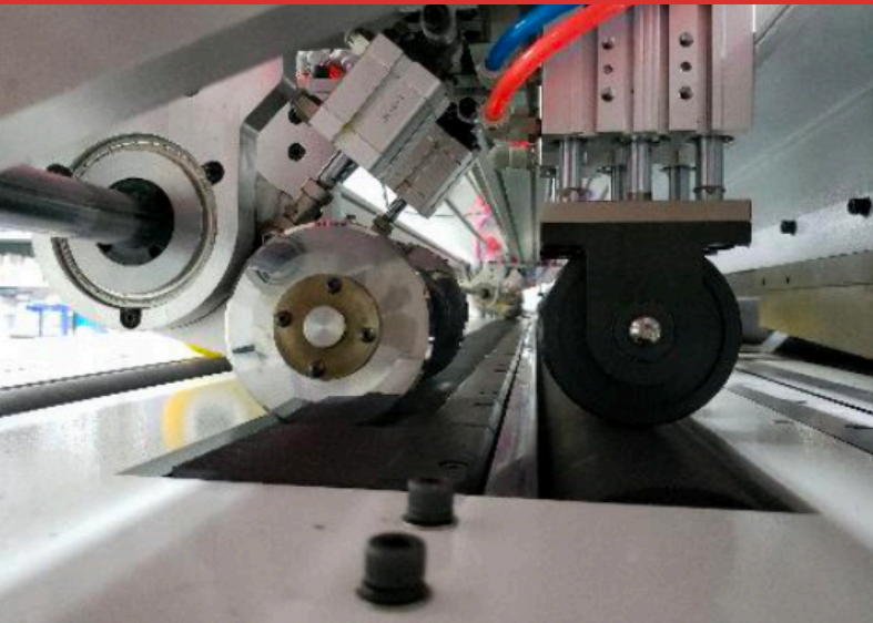
Schlitzmesser
